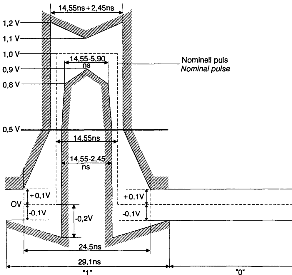
Figur 4:1 Pulsmask vid 34368 kbit/s
